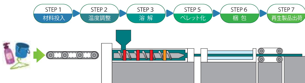
押出機
